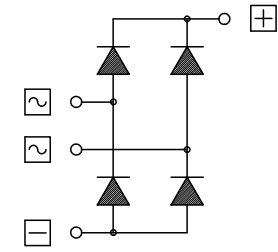
結線図
