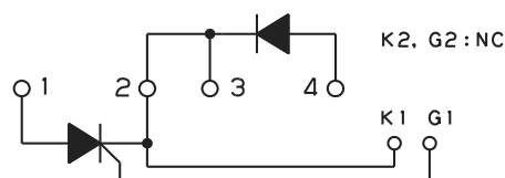
回路構成 Circuit Schema
