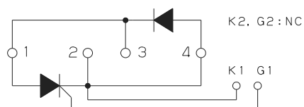
回路構成 Circuit Schema
