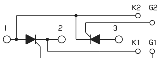
回路構成 Circuit Schema
