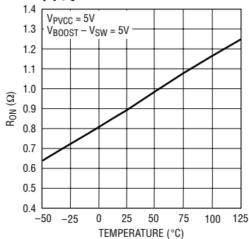
驱动器 R_{ON} 与温度关系 曲线
