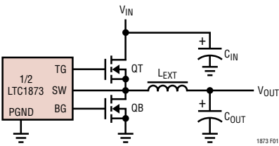
图 1：同步降压式变换器结构
