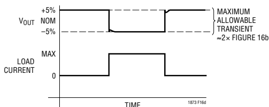
图 16d：设置稳压器——瞬态响应
