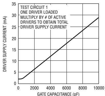
MOSFET 驱动器电源电流 与栅极电容关系曲线
