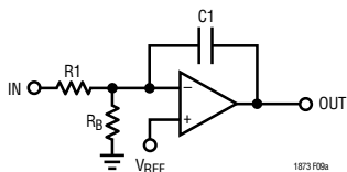
图 9a：类型 1 反馈环路中放大器接线图
