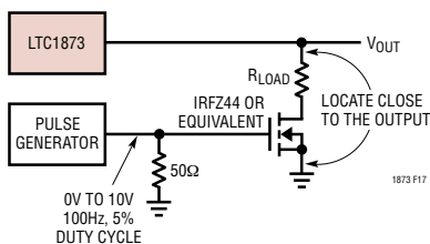
图 17：瞬态负载发生器
