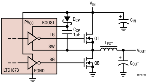
图 2：TG 驱动器的浮动电源
