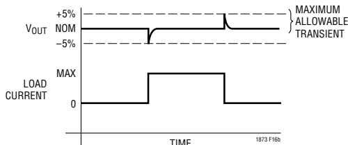
图 16b：标准稳压器——瞬态响应
