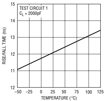
驱动器上升/下降时间与温度 关系曲线
