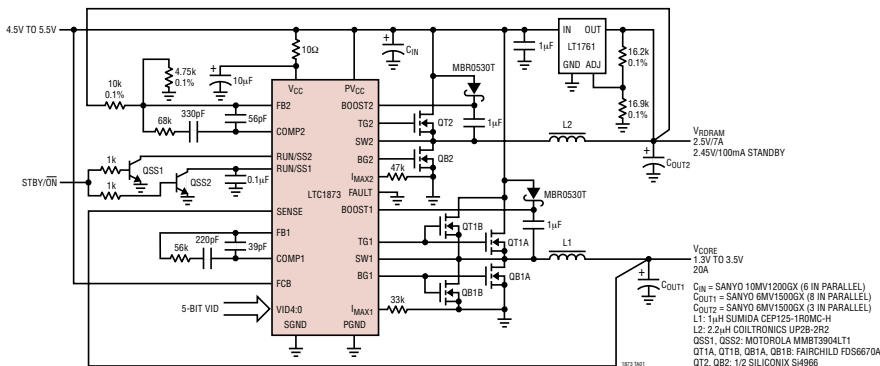
具有 RDRAM 维持功能的低成本台式计算机 CPU 用电源
