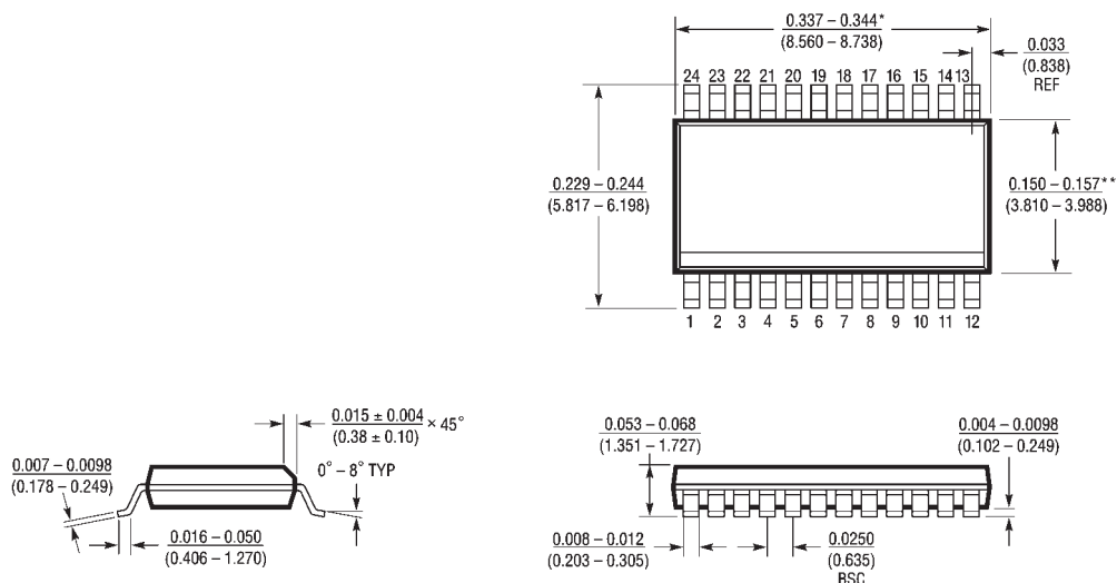
GN 封装 24 引脚塑料 SSOP 封装 (宽 .150 英寸) (参考 LTC DWG # 05-08-1641)
