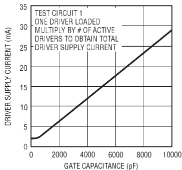
MOSFET 驱动器电源电流与门极电容关系曲线
