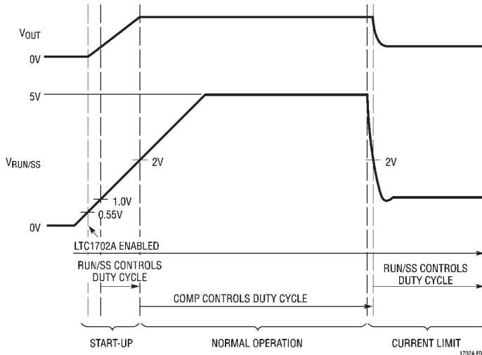
图 4：启动和限流时的软启动
