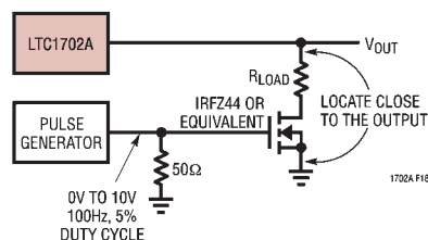
图 18：瞬态负载发生器
