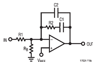
图10a：类型2放大器接线图
