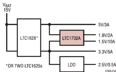
图 14：两步变换框图
