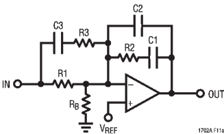
图 11a：类型 3 环路放大器接线图
