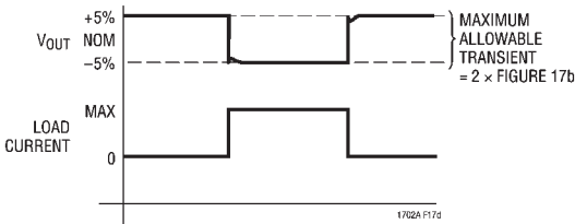
图 17d：设置稳压器——瞬态响应
