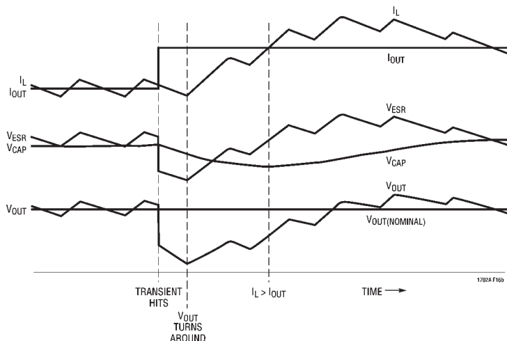
图 16b：瞬态恢复曲线
