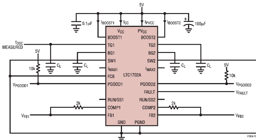
测试电路 1
