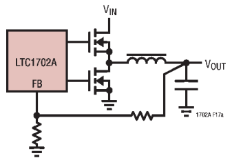
图 17a：标准稳压器
