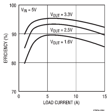
图 15：LTC1702A 典型效率曲线
