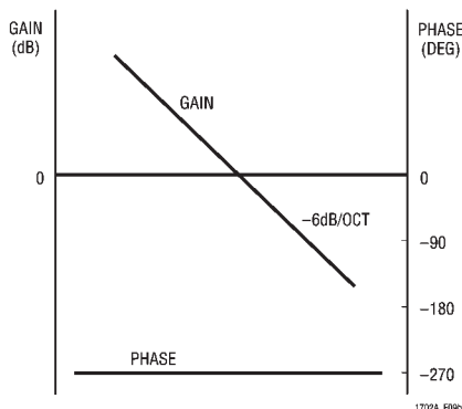
图9b：类型1放大器的传递函数
