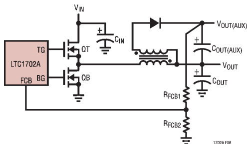
图 13：用 FCB 引脚调整辅助输出
