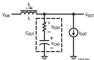
图 16a：电容器寄生效应影响 瞬态恢复时间
