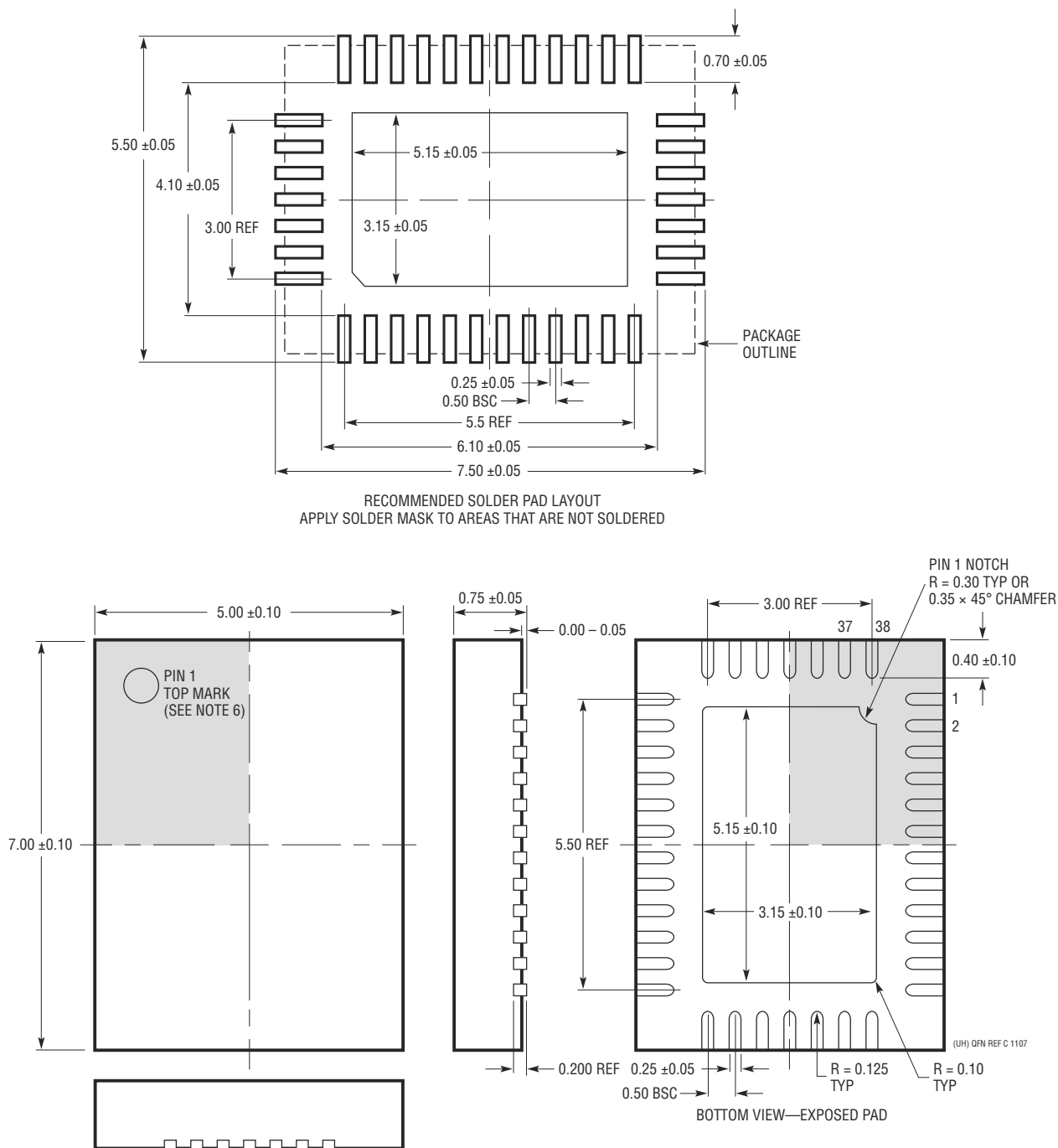
UHF 封装 38 引脚塑料 QFN (5mm × 7mm) (参考 LTC DWG # 05-08-1701 Rev C)
