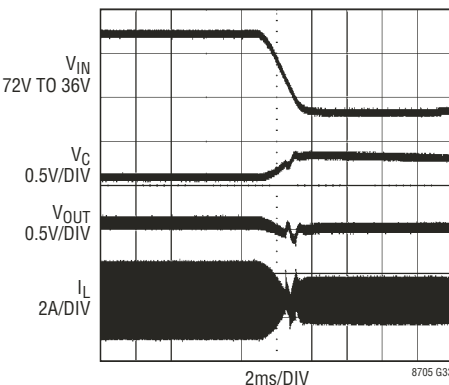
输入电压瞬变 (图 14)
