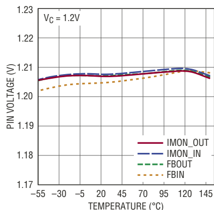
反馈电压
