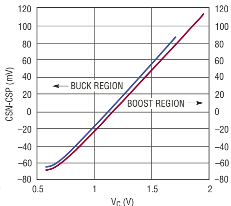
最小占空比下的电感电流 检测电压
