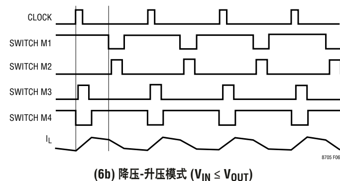
图 6：降压-升压区
