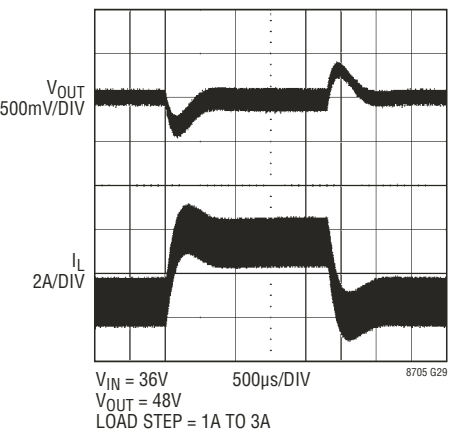
负载阶跃 (图 14)
