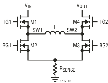
图 3：输出开关的简化示意图
