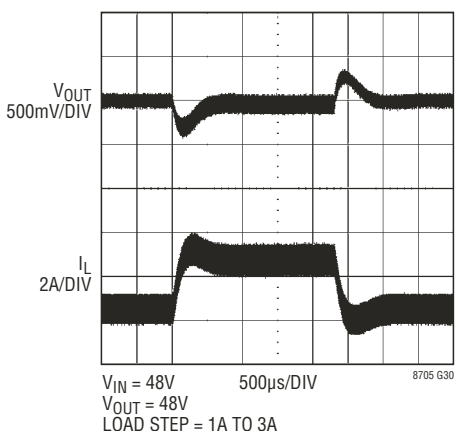
负载阶跃 (图 14)
