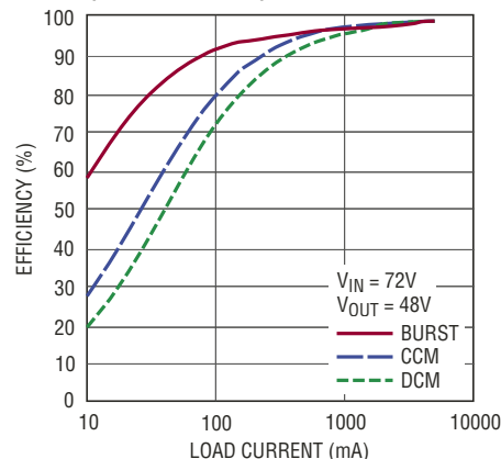
效率与输出电流的关系 (降压区 - 图 14)
