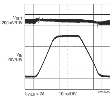
输入瞬变 (4V 至 80V)
