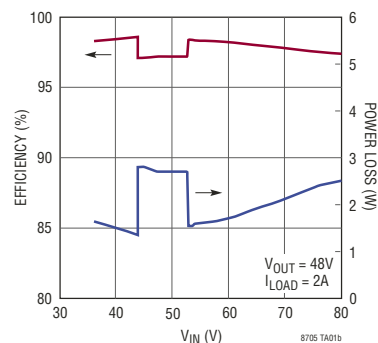
效率与功率损耗的关系
