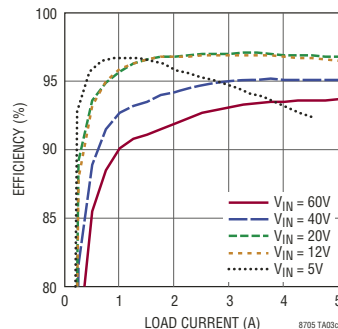
效率与输出电流的关系
