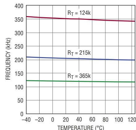
振荡器频率
