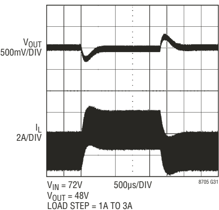
负载阶跃 (图 14)
