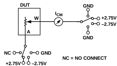
图42. 公共漏电流
