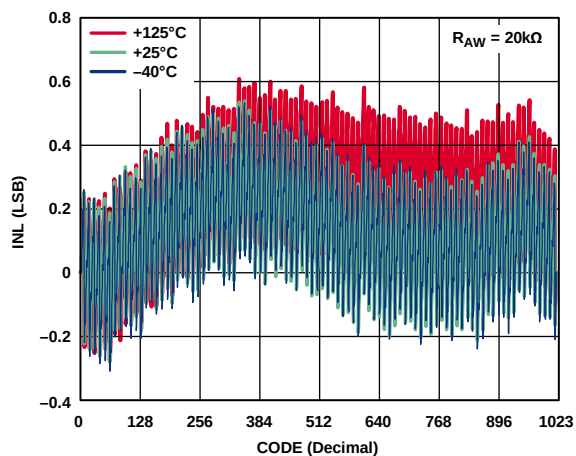
图6. R-Perf模式下R-INL与代码和温度的关系(AD5272)
