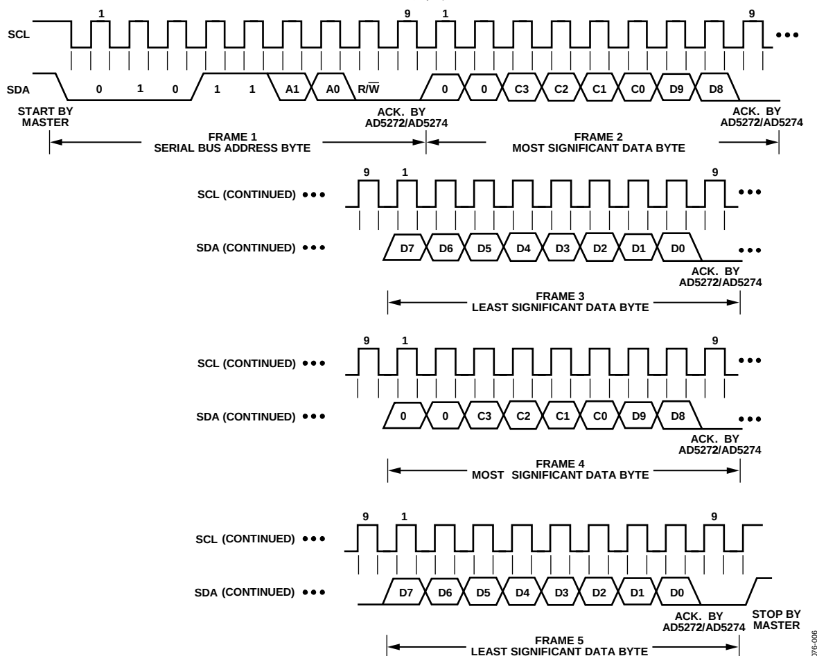
图44. 多次写入
