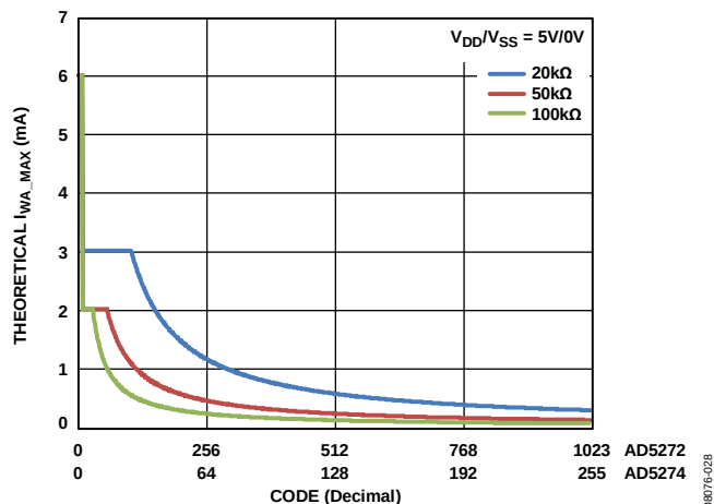
图27. 最大理论电流与代码的关系
