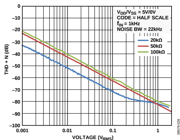
图33. THD + N与幅度的关系
