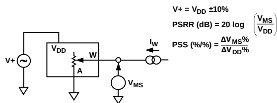
图40. 电源灵敏度( PSS , PSRR )
