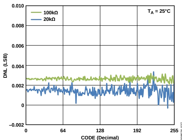
图22. 正常模式下R-DNL与代码和标称电阻的关系(AD5274)
