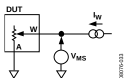
图38. 电阻位置非线性误差 (可变电阻器操作; R\text{-INL} , R\text{-DNL} )
