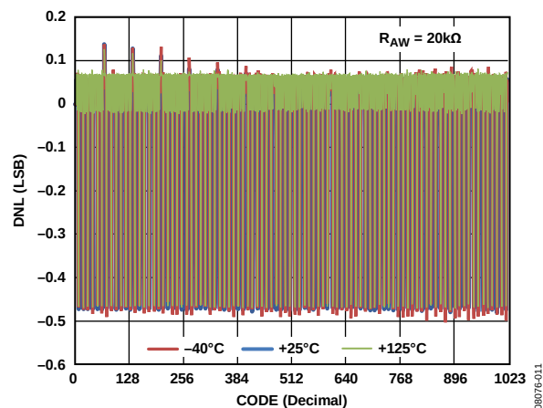
图7. R-Perf模式下R-DNL与代码和温度的关系(AD5272)
