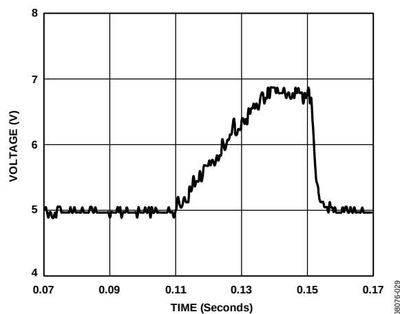
图36.写入熔丝时的 V_{EXT\_CAP} 波形
