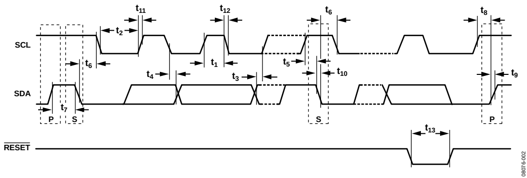
图3. 双线式串行接口时序图
