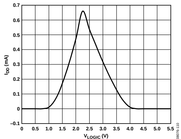
图23. 电源电流( I_{DD} )与数字输入电压的关系
