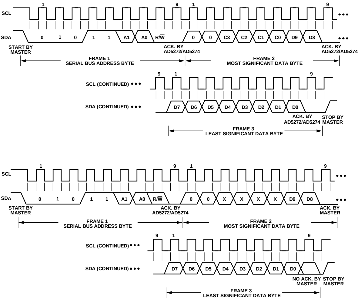
图45. 读命令
