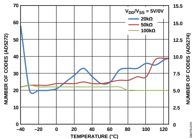
图35. 最大代码损失与电源范围的关系
