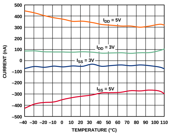
图20. 电源电流( I_{DD} , I_{SS} )与温度的关系
