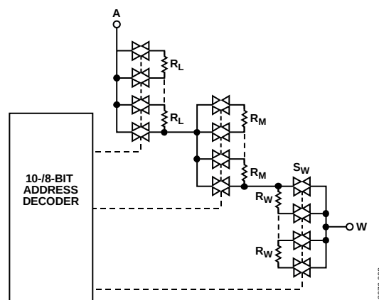
图46. RDAC电路示意图
