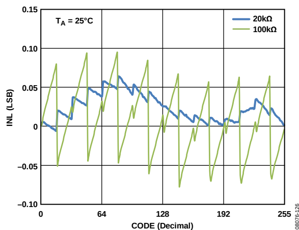
图21. 正常模式下R-INL与代码和标称电阻的关系(AD5274)
