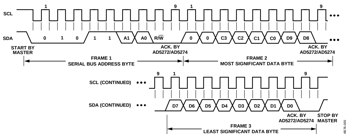
图43. 写命令
