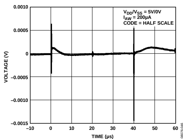
图34. 数字馈通
