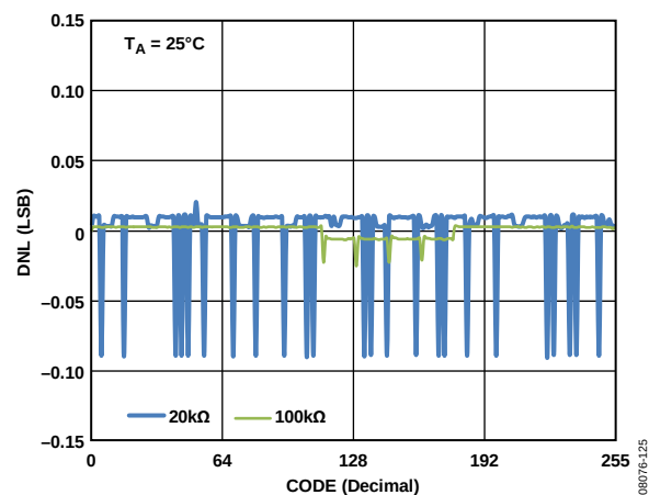
图17. R-Perf模式下R-DNL与代码和标称电阻的关系(AD5274)
