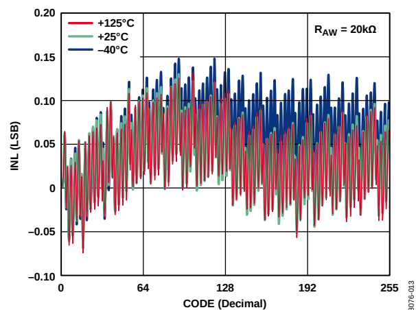
图13. R-Perf模式下R-INL与代码和温度的关系(AD5274)
