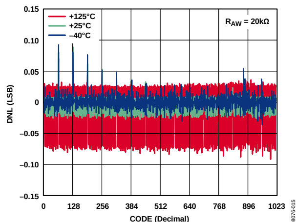
图12. 正常模式下R-DNL与代码和温度的关系(AD5272)
