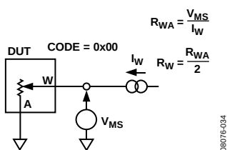
图39. 游标电阻
