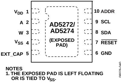
图5. LFCSP引脚配置
