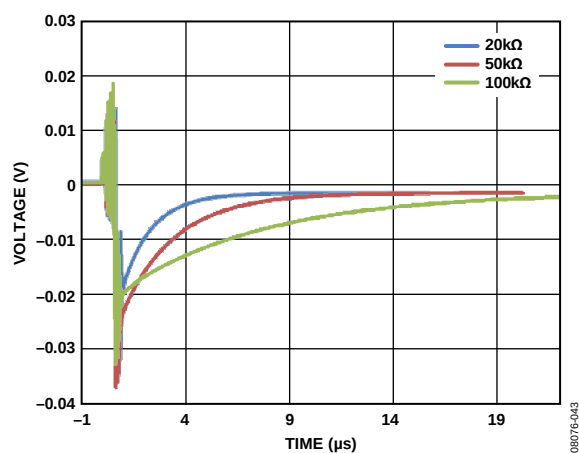
图31. 最大毛刺能量
