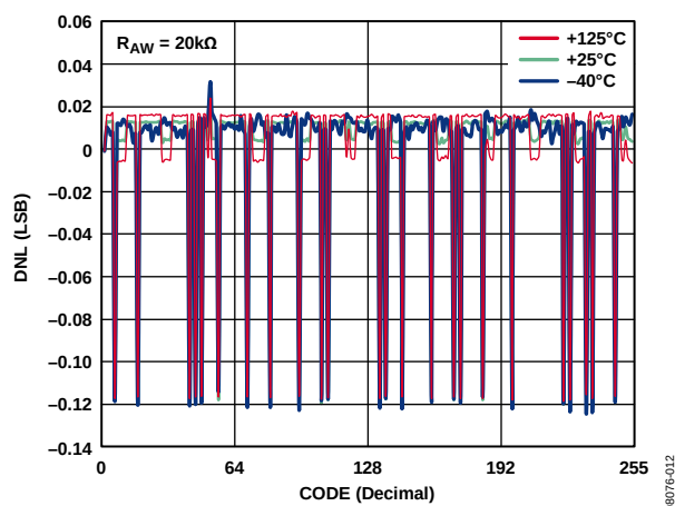
图14. R-Perf模式下R-DNL与代码和温度的关系(AD5274)
