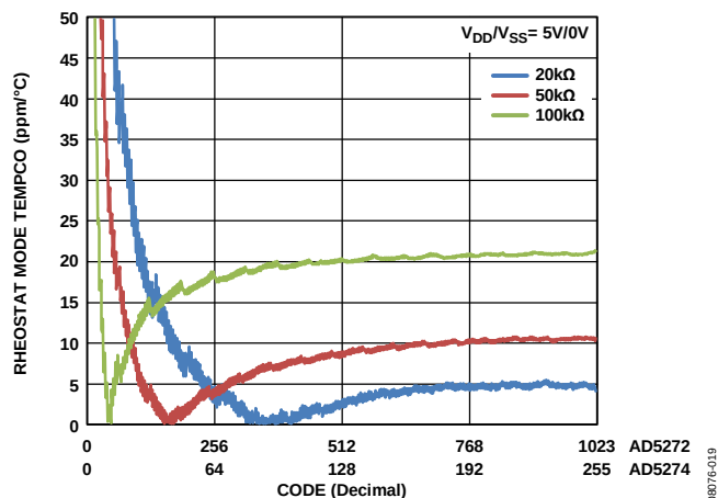
图24. \text{Tempco } \Delta R_{WA}/\Delta T 与代码的关系
