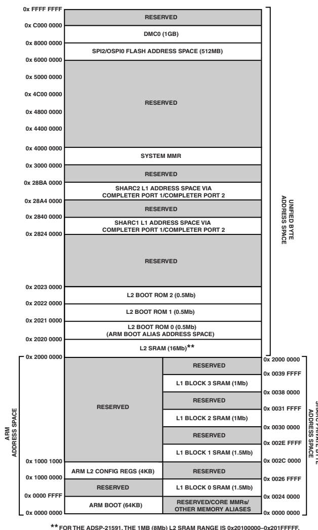
Figure 5. ADSP-2159x/ADSP-SC59x Memory Map
