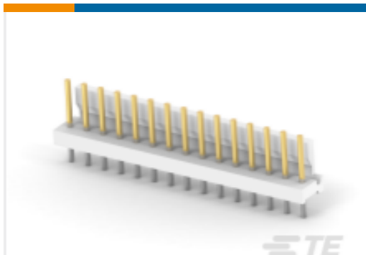
TE 产品编号 4-644760-5 15P MTA156 HDR ASSY FL ST LF
