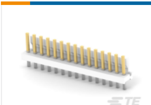
TE 产品编号 4-644759-5 15P MTA156 HDR ASSY STR LF
