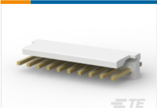
TE 产品编号 4-641208-0 10P MTA156 HDR ASSY FL ST LF
