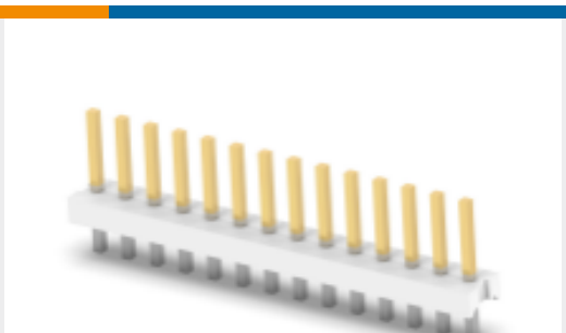
TE 产品编号 4-644756-4 14P MTA156 HDR ASSY STR AU LF
