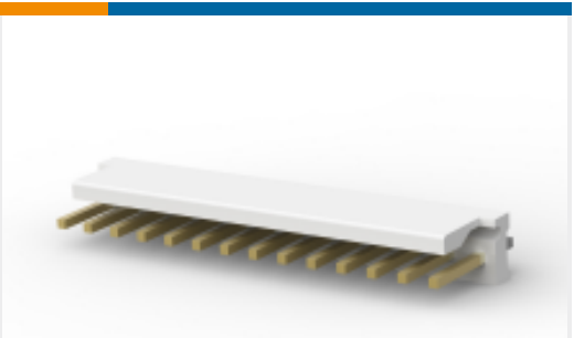
TE 产品编号 4-641208-4 14P MTA156 HDR ASSY FL ST LF
