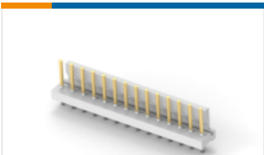
TE 产品编号 4-641209-4 14P MTA156 HDR ASSY FL ST LF
