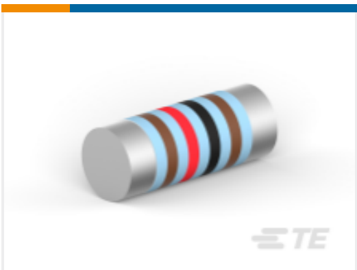
TE 产品编号4-1879283-0 MELF SMA 56K 1% 50PPM 1W 0207
