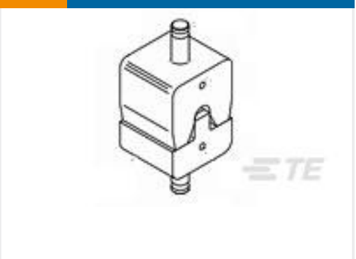
TE 产品编号48861-1 HYP8/10 PLASTI-GRIP/10 2AWG DIE SET
