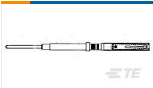
TE 产品编号1-211431-8 SKT CONTACT ASSY, SZ 22
