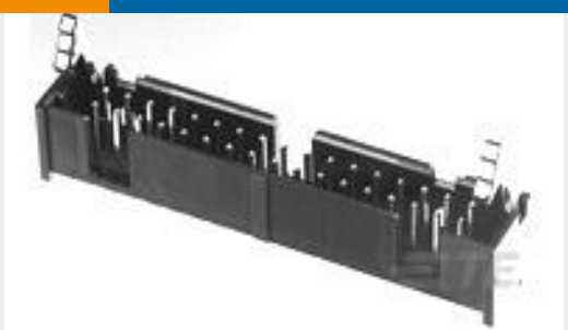
TE 产品编号1-1761608-3 IDC LOW PRO HDR 40P VERT SHT L
