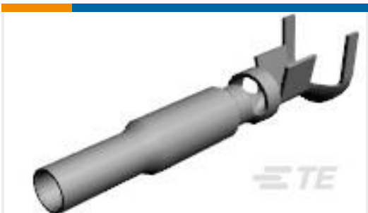
TE 产品编号1-770249-0 UMNL II SOK SN/AUNI/PHBZ LP
