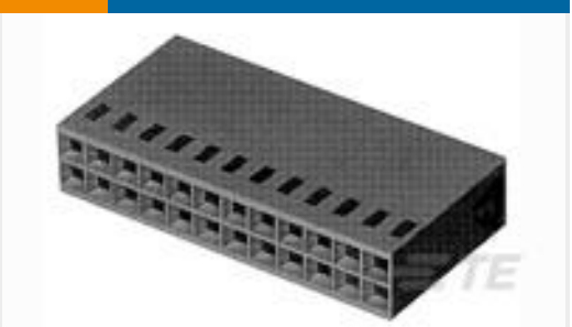
TE 产品编号1-87456-2 16 MODIV HSG DR MRKD .100CL
