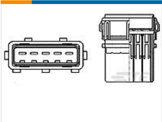
TE 产品编号444208-1 ASSY 5 POSN JPT TAB
