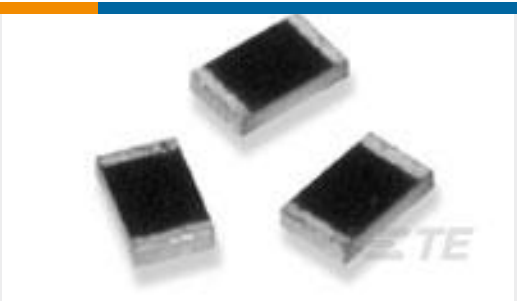
TE 产品编号1625868-7 RP 2A 0.25W 215K 0.1% 25PPM 1K RL
