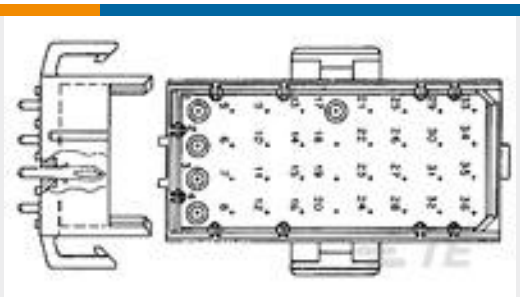
TE 产品编号2-640499-4 04P MR HDR ASSY VO RED LF
