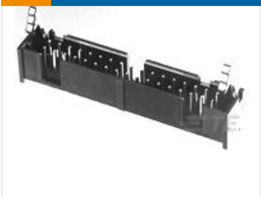
TE 产品编号2-1761608-8 IDC LOW PRO HDR 24P VERT SHT L
