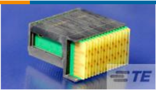
TE 产品编号 1410139-1 MULTIGIG RT T2 .8" DC DF F-RGT
