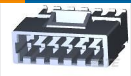
TE 产品编号3-641522-6 06P MTA156 POST CON ASSY ORNG
