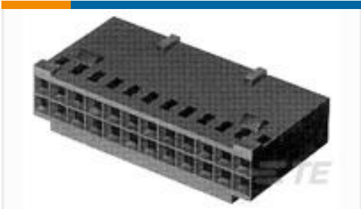
TE 产品编号 3-88179-8 030 HOUSING FFC RCPT DR 100CL
