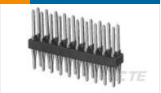
TE 产品编号5-103233-2 06 MODII HDR DRST UNSHRD A/PIN
