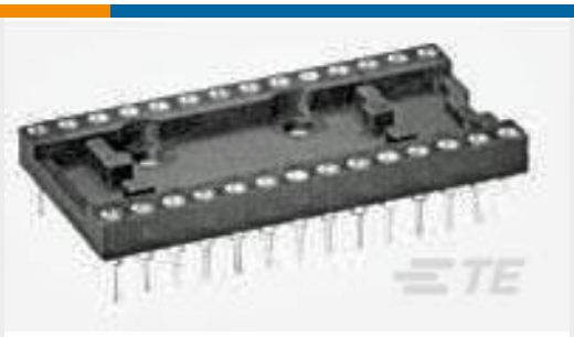
TE 产品编号2-1571551-6 520-AG11D-ESL-LF=500 DIP,GF/SN
