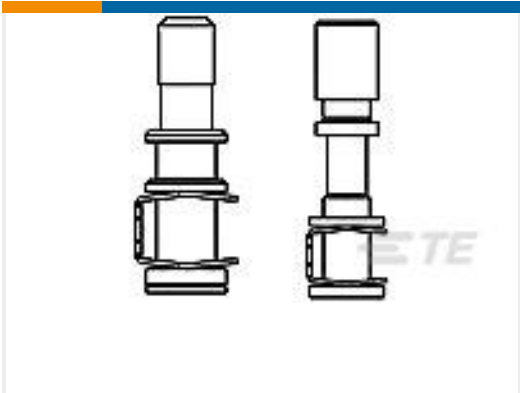
TE 产品编号1355532-3 LWL INSERT
