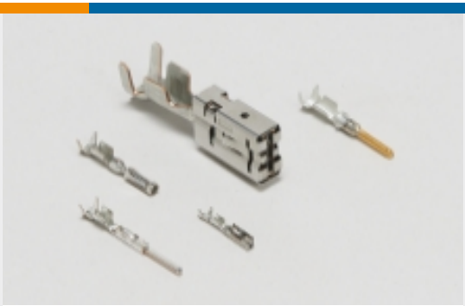
汽车端子(31)
