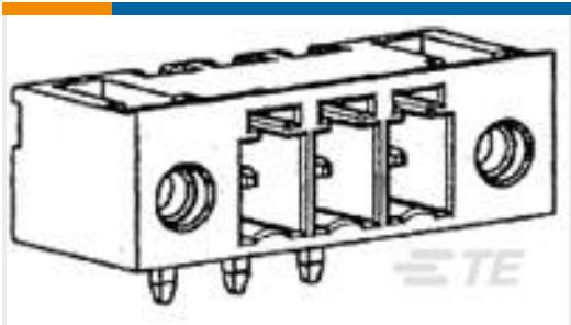
TE 产品编号1-284539-2 12 POS TERMINAL-BLOK 900 W.S.F. 3,
