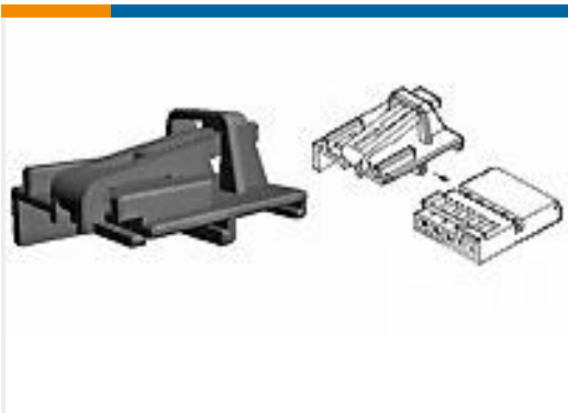
TE 产品编号1418776-2 COVER,MQS,5 POS.
