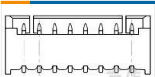
TE 产品编号1-1734829-0 1.25 WTB HDR DIP, 10 POS
