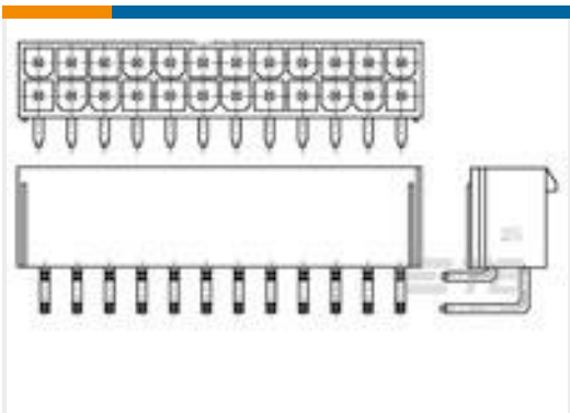
TE 产品编号2-1586042-0 20P VAL-U-LOK R/A HDR V0
