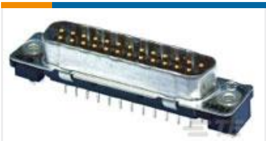
TE 产品编号1-338311-2 25POS.HD20 PLUG ASS
