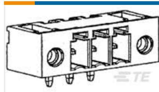
TE 产品编号1-796866-0 10POS TERMI-BLOK HDR RT ANGLE
