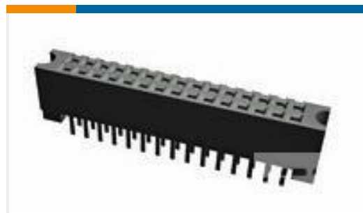
TE 产品编号 5-534972-1 30 MODII VRT 2PC DR CE 100CL, RoHS
