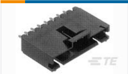
TE 产品编号9-1437539-1 828-AG11D-ES=SOCKET ASSY
