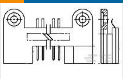
TE 产品编号583580-1 BOX PIN 50 POS. 100 C/L
