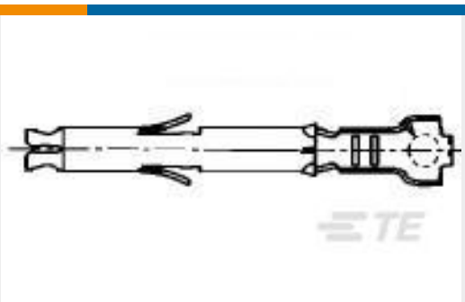
TE 产品编号170366-4 MINI UNIVERSAL M-N-L SOCKET LP
