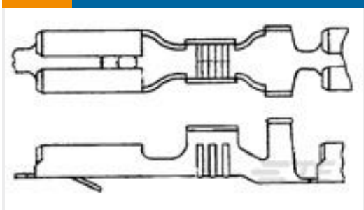
TE 产品编号170042-1 FF 110 REC 20-16AWG BR
