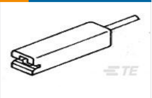
TE 产品编号1-480417-0 110 FASTON HSG.,REC.,1 POS, NATRUAL
