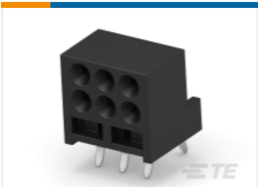
TE 产品编号1376962-1 FAN MOTOR CONN HDR ASSY T/E
