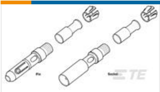
TE 产品编号201143-1 MIN PIN
