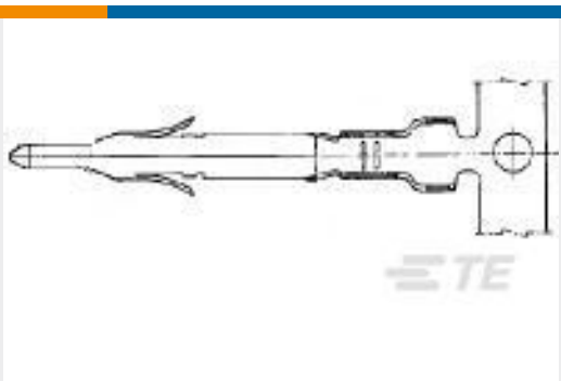
TE 产品编号170363-3 MINI UNIVERSAL M-N-L PIN LP
