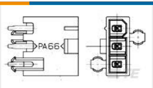
TE 产品编号2029054-3 3P VAL-U-LOK SR HDR SN V2 W/DH
