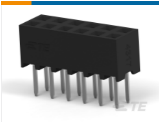
TE 产品编号1-2314812-2 12P, 2MM, B-B, REC, DRV T, 2.0, 0.1AU, TB, W/CAP
