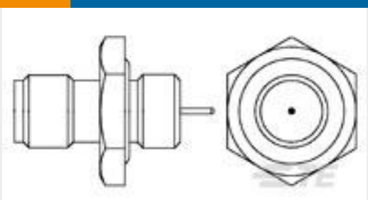
TE 产品编号1053137-1 2058 3100 00
