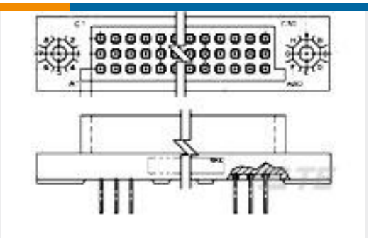
TE 产品编号532786-5 3 ROW BOX RECP 165 POS 100 C/L
