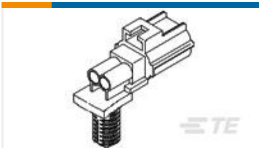
TE 产品编号184176-1 2 POS. END CAP ASSY., KEY A
