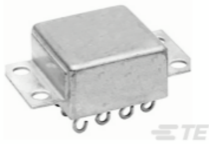
TE 产品编号 1617086-8 3SBM1086A2 = M39016/36-003M
